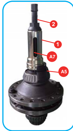
Remove the differential rear bearing: 拆卸差速器後培林
