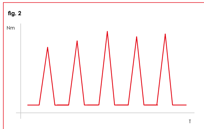
Diagramma della coppia di serraggio in un avvitatore a massa battente. Diagram of the tightening torque in an impact wrench. Diagramme du couple de serrage dans une visseuse à masse battante. Diagrama de la par de torsión de cierre en un atornillador percutor.
