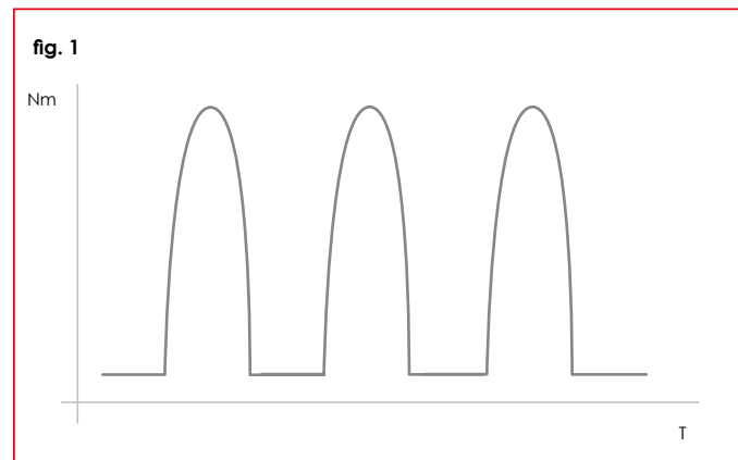
Diagramma della coppia di serraggio in un avvitatore idraulico ad impulsi. Diagram of the tightening torque in a hydraulic pulse wrench. Diagramme du couple de serrage dans une visseuse hydraulique à impulsions. Diagrama de la par de torsión de cierre en un atornillador hidráulico de impulsos.
